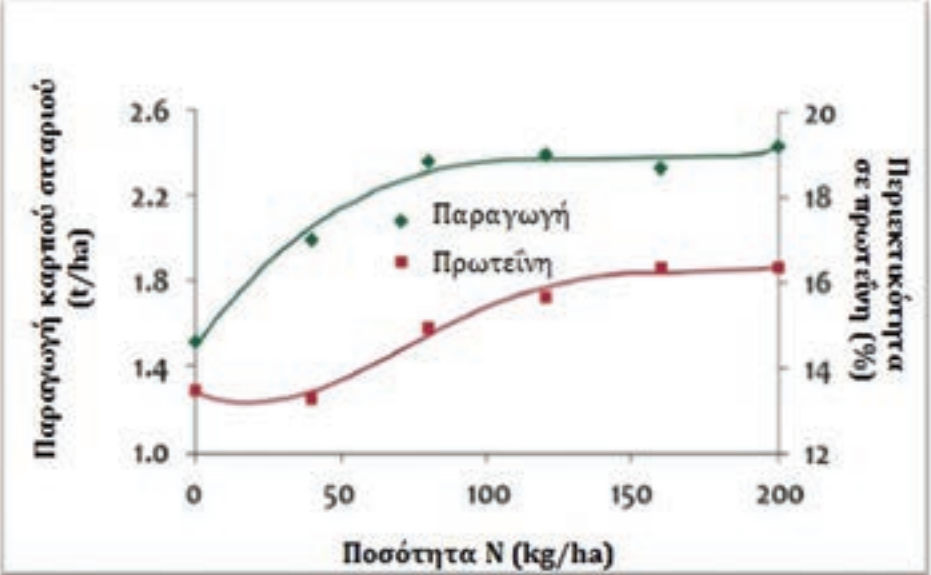
Σχήμα 2: Η σχέση μεταξύ της αναμενόμενης παραγωγής καρπού στα σιτηρά και της περιεκτικότητάς τους σε πρωτεΐνη συνδέεται με την ποσότητα του αζώτου.
