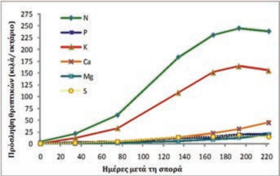
Σχήμα 1: Ο ρυθμός πρόσληψης των θρεπτικών στοιχείων από την καλλιέργεια σιταριού επηρεάζεται ανάλογα με το στάδιο ανάπτυξής της, δηλαδή τις ημέρες μετά τη σπορά.
