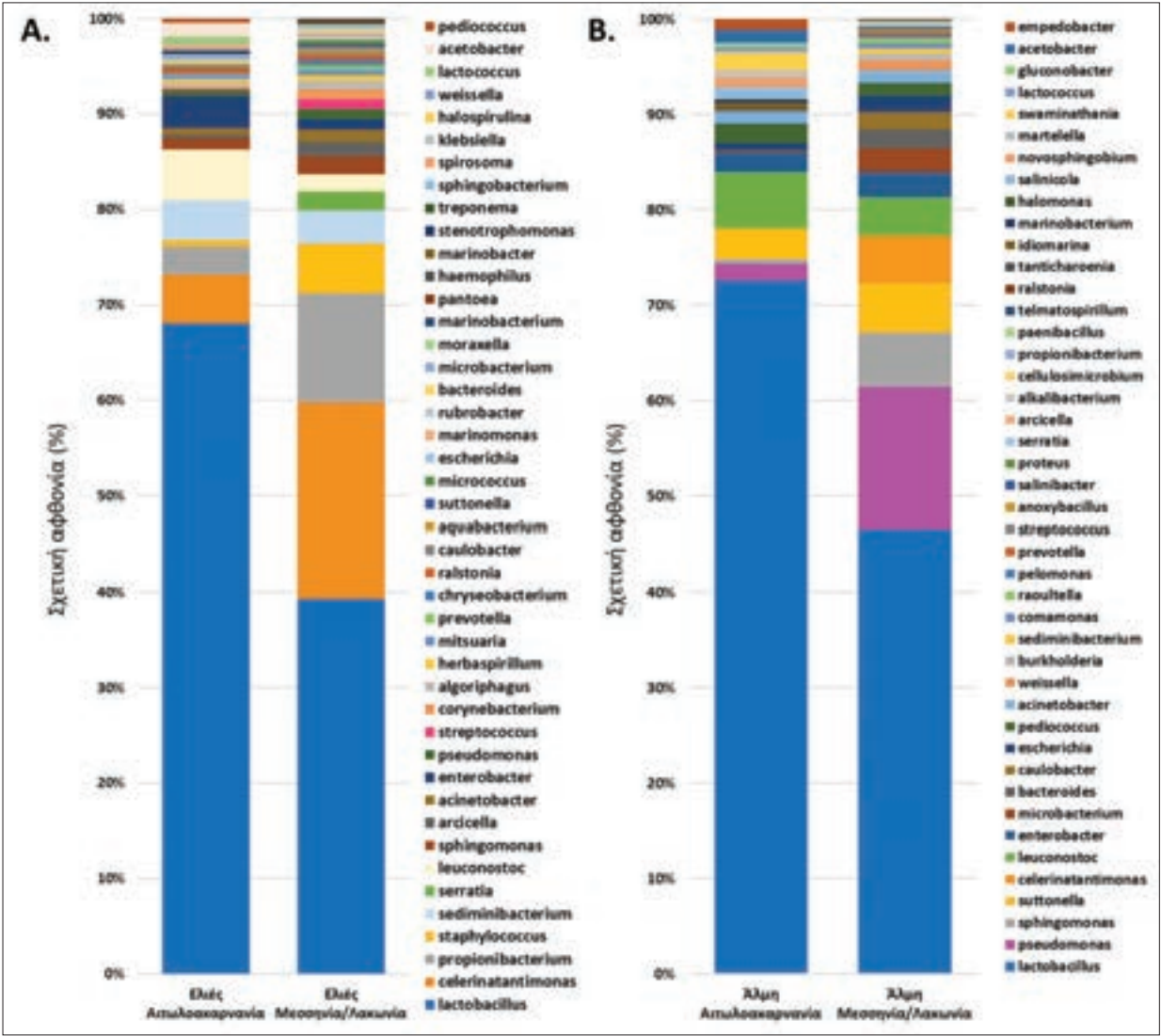
Γράφημα 1: Μέση τιμή σχετικής αφθονίας (%) των κυρίαρχων γενών βακτηρίων που ταυτοποιήθηκαν μέσω της 16S rRNA μεταγονιδιωματικής ανάλυσης σε δείγματα καρπού ελιάς (Α) και άλμης (Β) της φυσικής μαύρης ελιάς της ποικιλίας Καλαμών από τους Νομούς Μεσσηνίας/Λακωνίας και τον Νομό Αιτωλοακαρνανίας.
