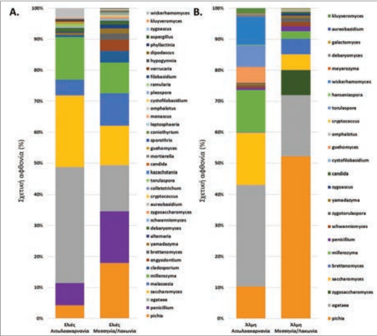
Γράφημα 2: Μέση τιμή σχετικής αφθονίας (%) των κυρίαρχων γενών ζυμών/μυκήτων που ταυτοποιήθηκαν μέσω της ITS μεταγονιδιωματικής ανάλυσης σε δείγματα καρπού ελιάς (Α) και άλμης (Β) της φυσικής μαύρης ελιάς της ποικιλίας Καλαμών από τους Νομούς Μεσσηνίας/Λακωνίας και τον Νομό Αιτωλοακαρνανίας.
