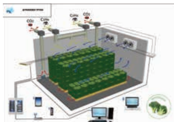
Σχηματική αναπαράσταση της «Δυναμικής Ψύξης».
